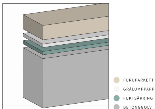
Montering på betongplatta med träbaserat flytande undergolv
