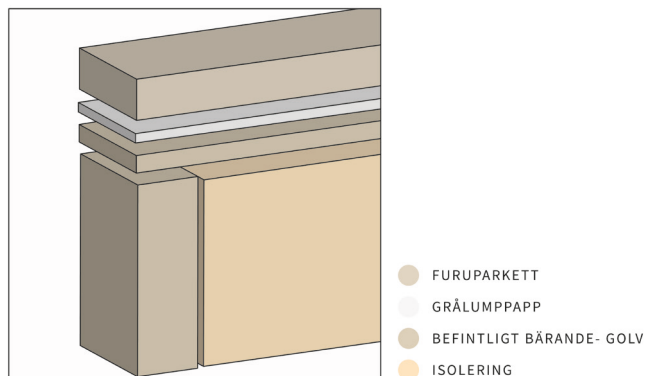
Befintligt undergolv
