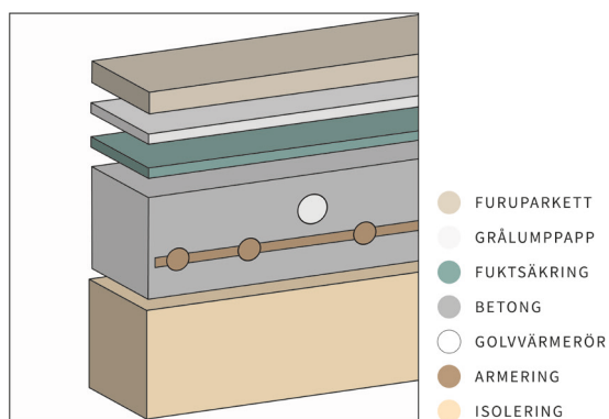
Betonggolv med ingjuten golvvärme
